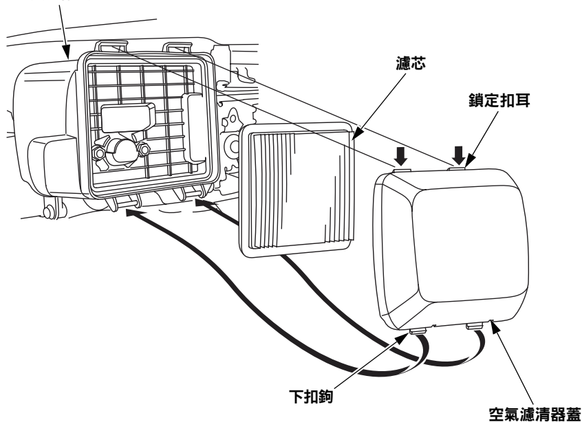
空氣濾清器殼
