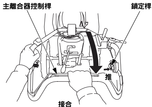
抓握位置 2
