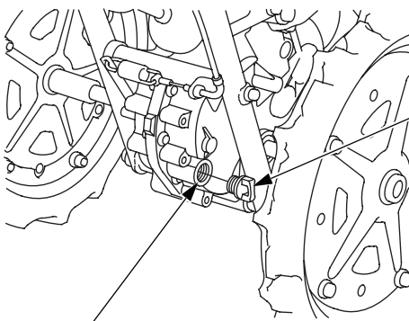
機油加油孔
